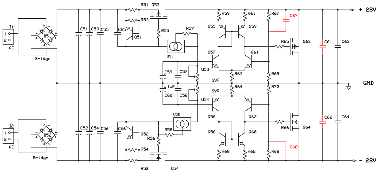
Euleit ULTIMA-Pre EU-01 MKII MOSFET SHUNT REGULATOR v2.2
