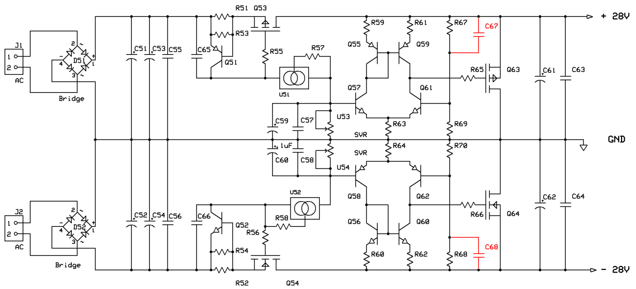
Euleit ULTIMA-Pre EU-01 MKII MOSFET SHUNT REGULATOR v2.1
