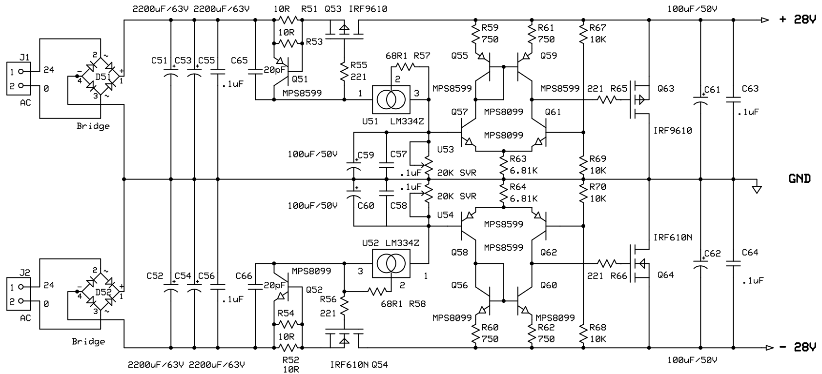
DZ ULTIMA-PRE MOSFET SHUNT REGULATOR
